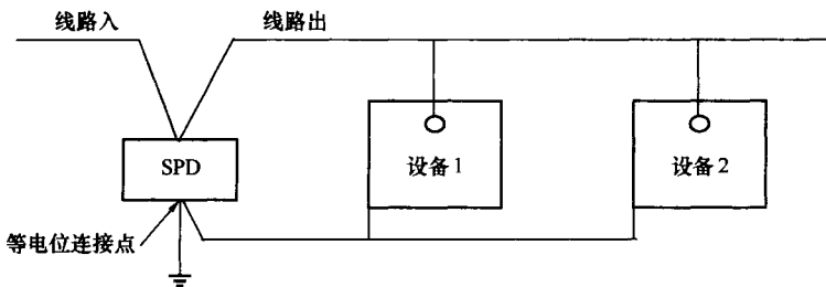
图 11 凯文接线法
