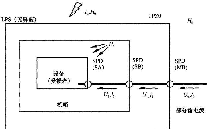
(d) 仅采用“协调配合的SPD防护”的LPMS ——对于传导浪涌 ( U_2 < U_0 和 I_2 < I_0 ), 设备得到防护; 但对于辐射磁场 ( H_0 ) 却无防护作用
